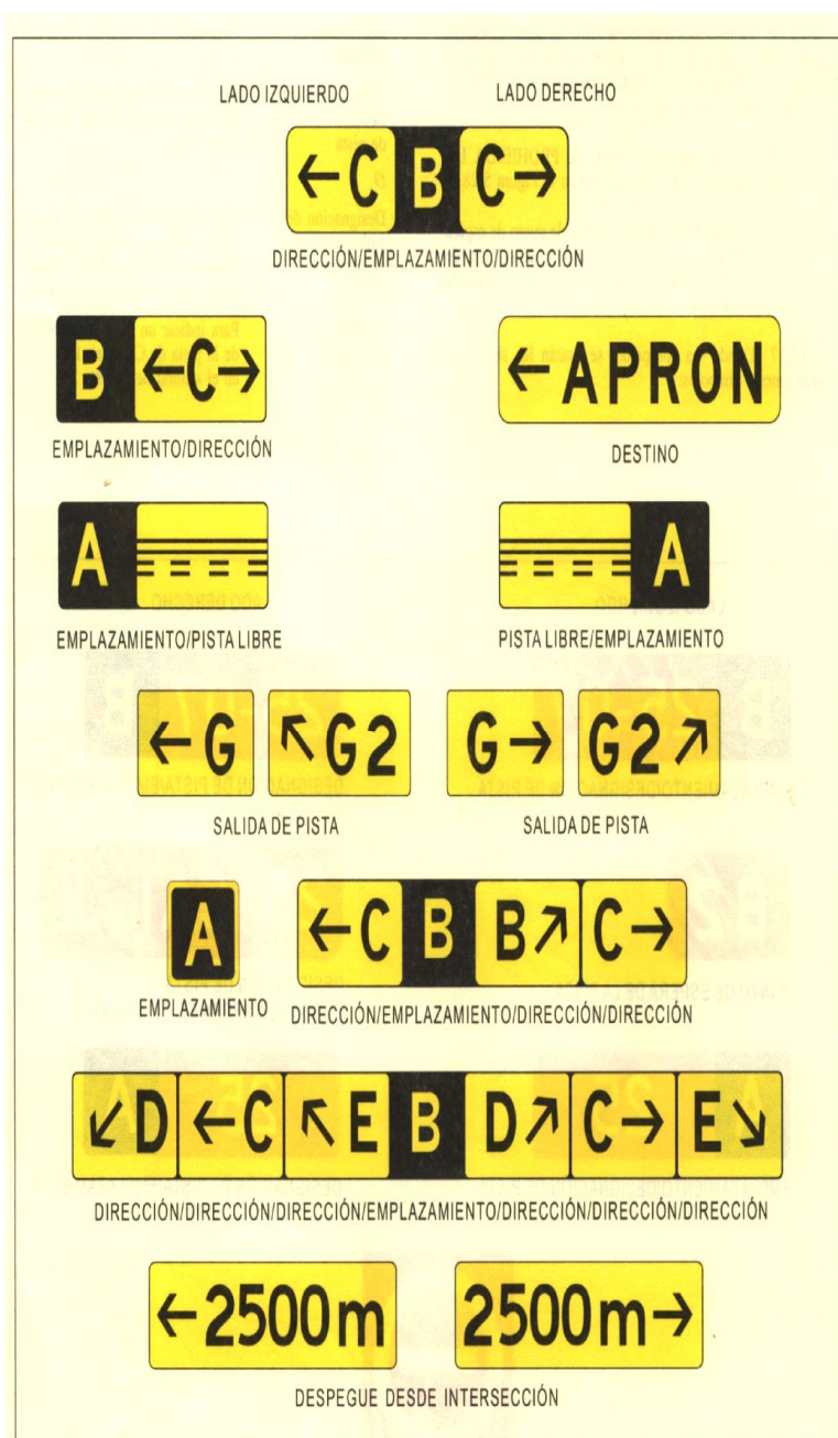
Figura 5-29. Letreos de información
