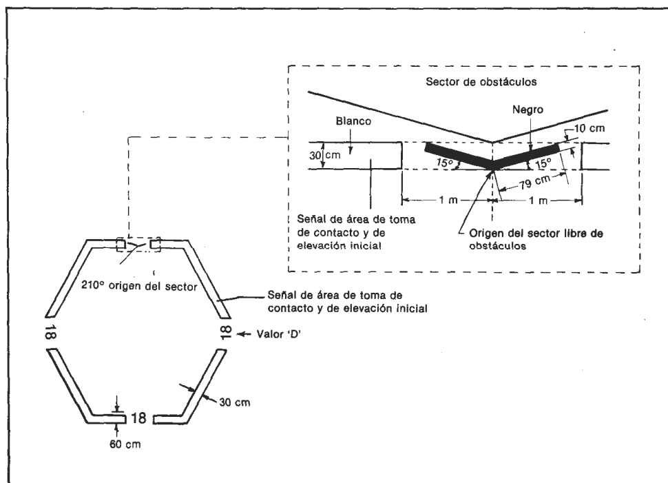
Figura 5-5H. Señal de sector despejado de obstáculos de heliplataforma
