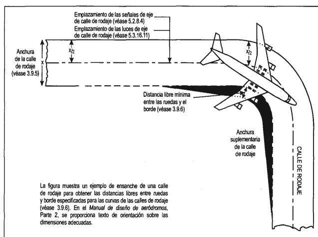
Figura 3 - 2. Curva de calle de rodaje
