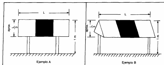
Figura 5-7H. Baliza de ruta de desplazamiento aéreo
