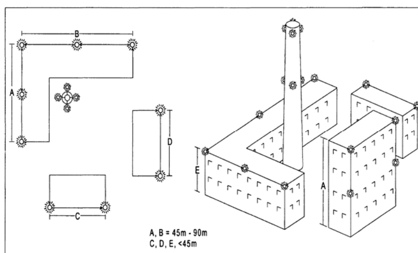
Figura 6-3. Iluminación de edificios
