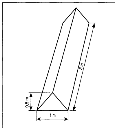
Figura 5 -32. Balizas delimitadoras
