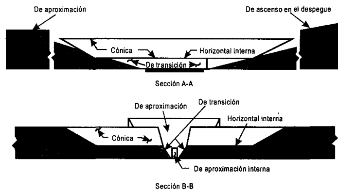
Continuación Figura 4 - 1. Superficies limitadoras de obstáculos
